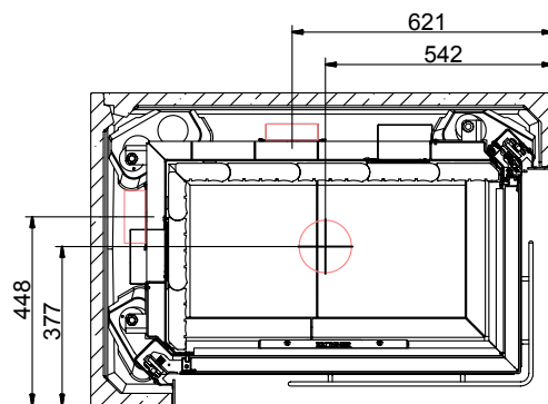
SCHNITT A-A
