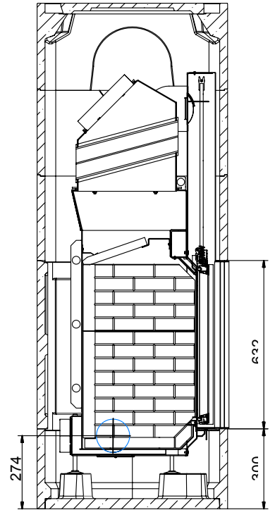
SCHNITT A-A
