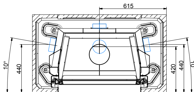
SCHNITT B-B
