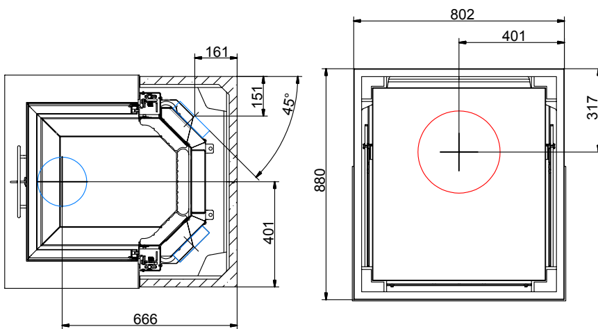
SCHNITT B-B
