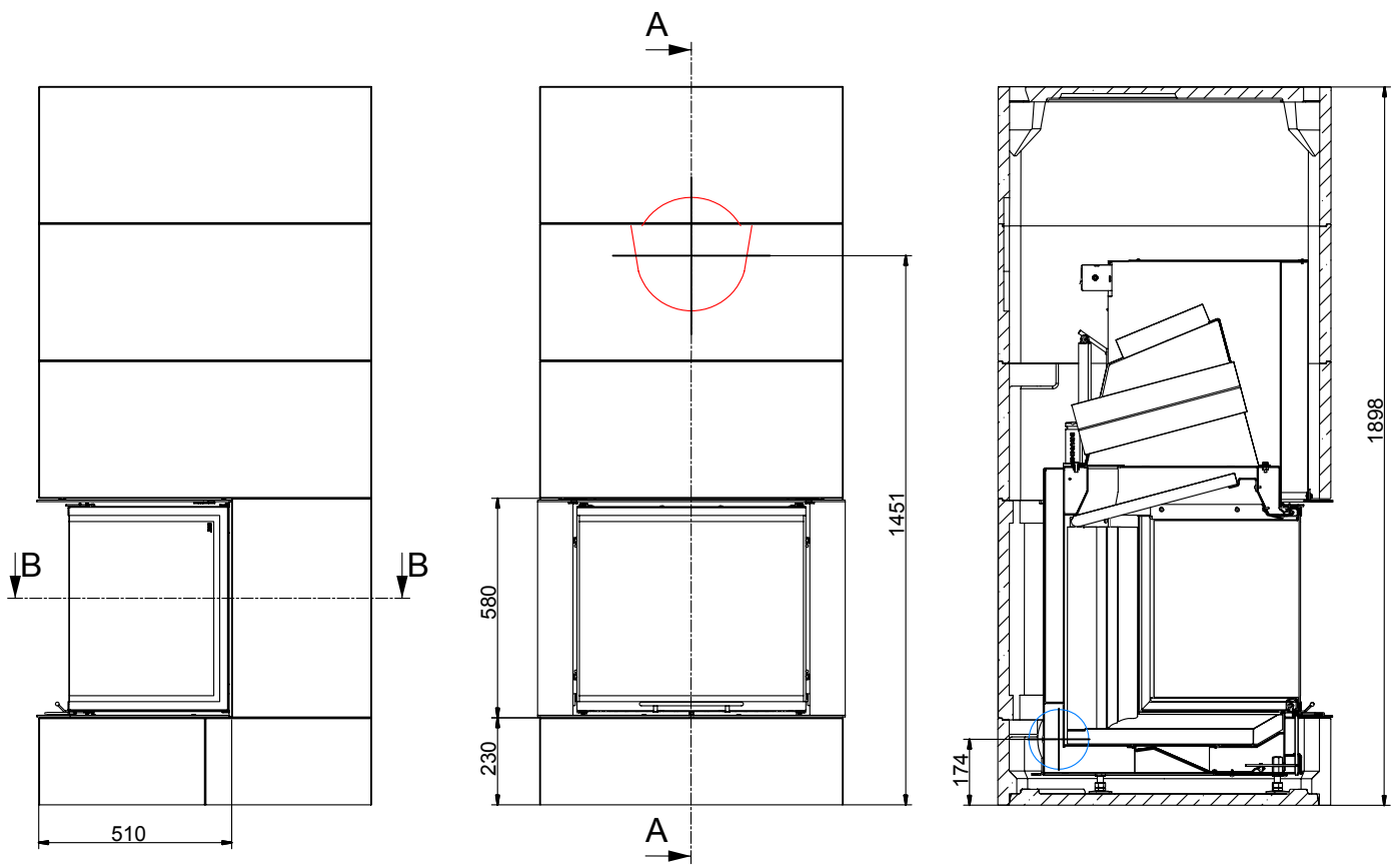
SCHNITT A-A
